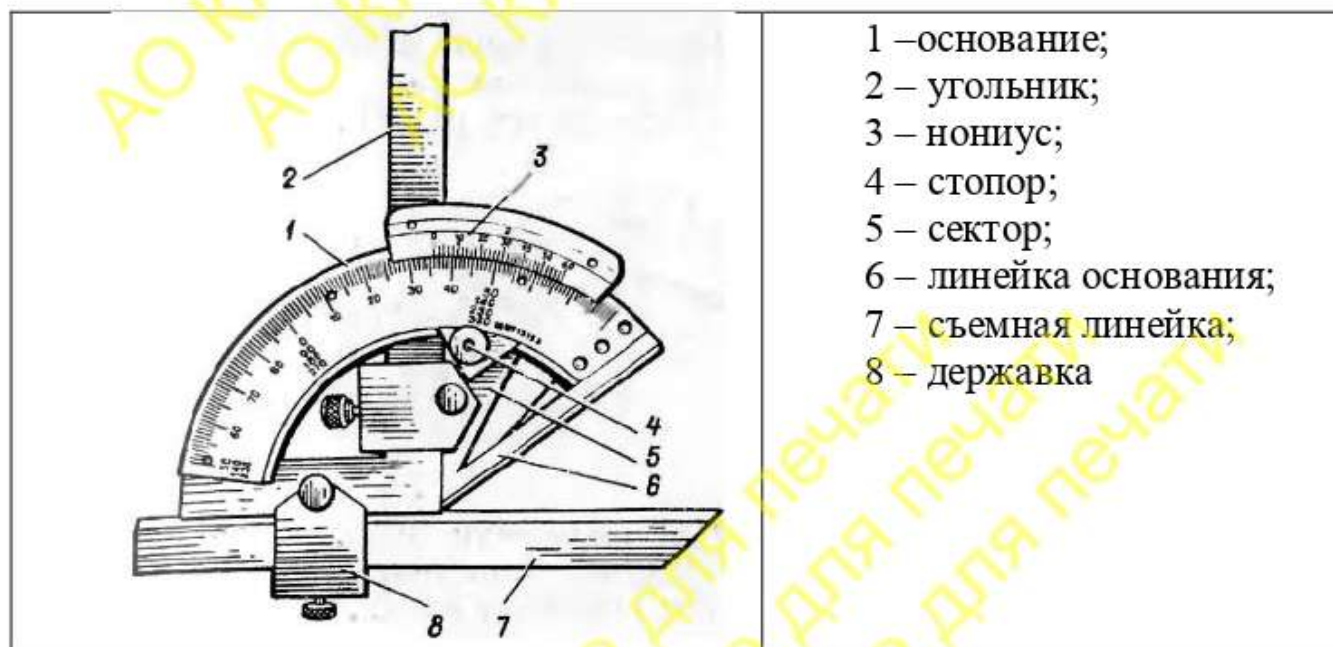
Рис. 2 – Схема угломера модификации УН-320
